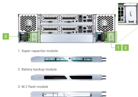
Модули Cache-to-Flash
